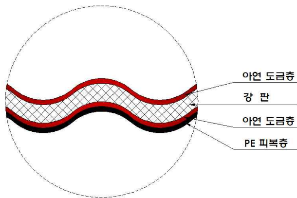
그림 1. 일반형 강관 및 유공관의 내면 피복 강판의 단면 모양
