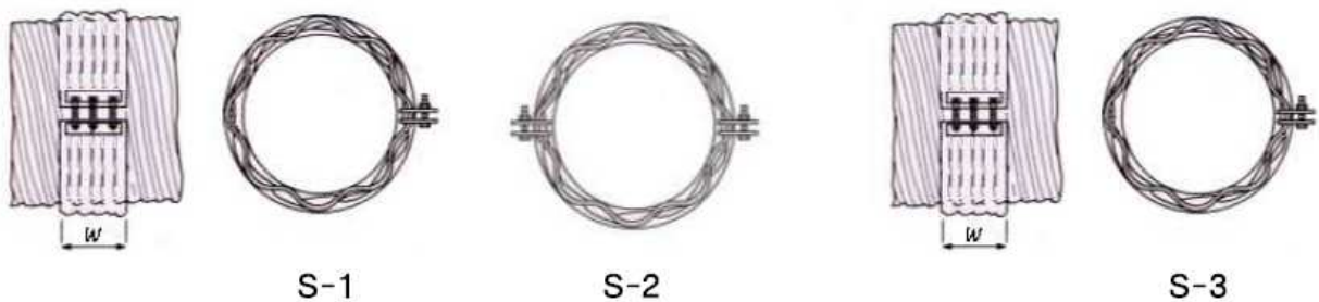
그림 7. 피복 커플링밴드의 모양
