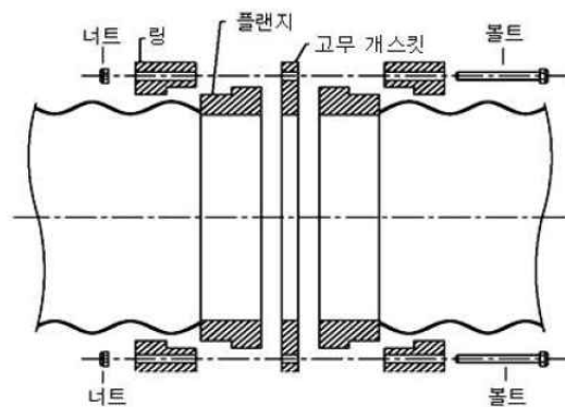
그림 8. PE 플랜지의 결합 구조
