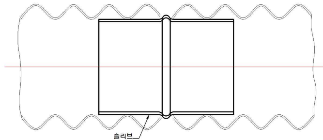
그림 6. 슬리브의 결합 구조
