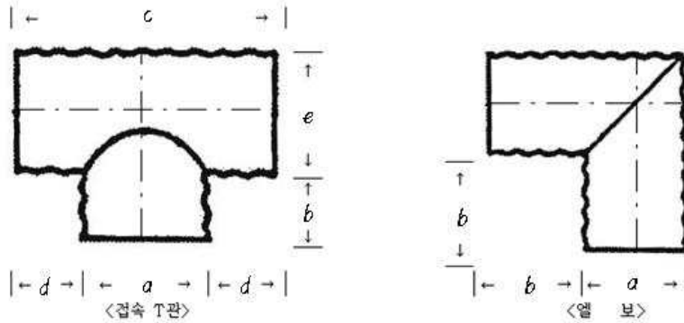
그림 11. 접속 T관 및 엘보의 구조
