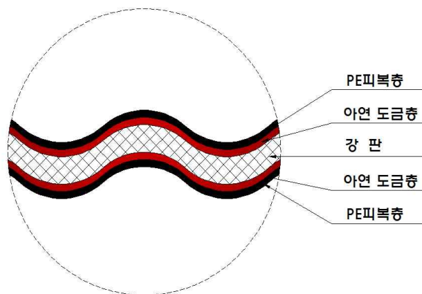
그림 2. 일반형 강관 및 유공관의 양면 피복 강판의 단면 모양
