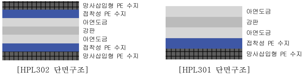
그림 3. 그물망 형태의 망사가 적층된 피복 강판의 단면 모양
